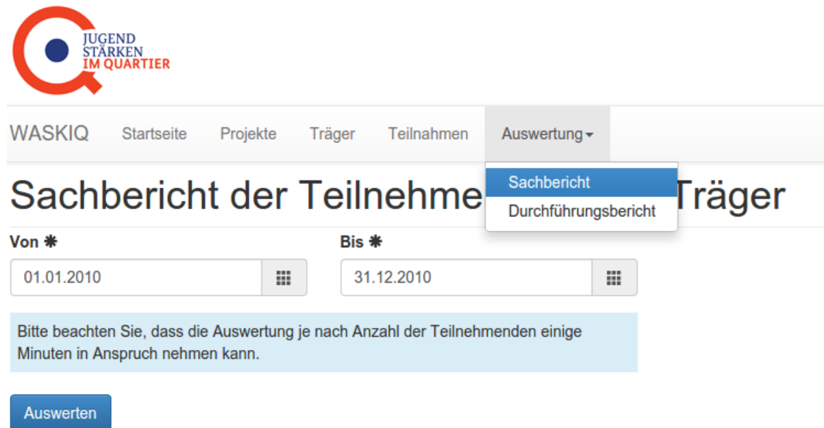
Abbildung 1.14: Screenshot: Auswertung
